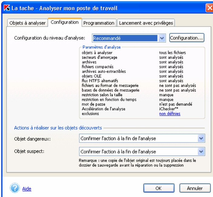
Illustration 20. Configuration de l'analyse à la demande
