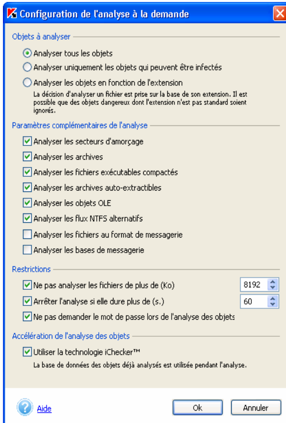
Illustration 21. Configuration détaillée de l'analyse à la demande
