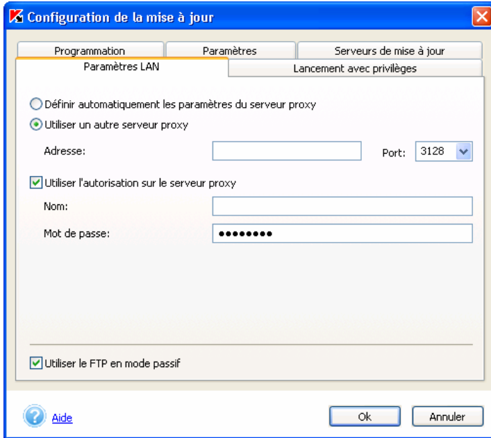
Illustration 13. Configuration des paramètres LAN
